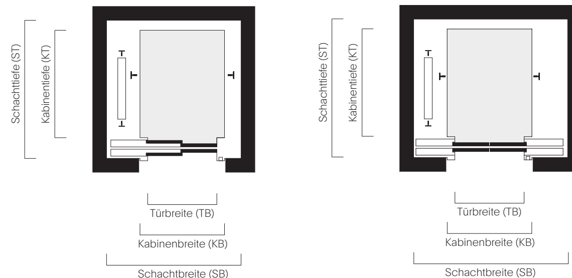
Grundriss
