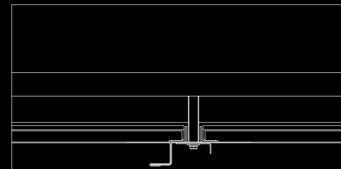
Horizontalschnitt Seitenwand, Handlaufseite. Handlaufauflager.
