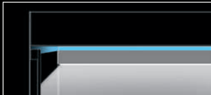
Vertikalschnitt LD8-LED-RGB-Lichtdecke. Funktionsschema Direkt-Indirektbeleuchtung. LED Neutralweiß, LED-RGB-Lichtsteuerung.
